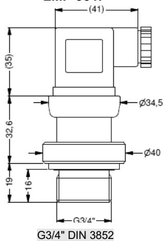
G3/4" DIN 3852
