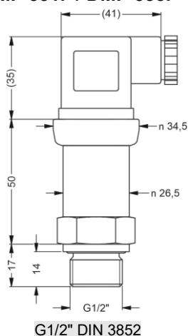
G1/2" DIN 3852
