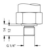
G1/4" DIN 3852
