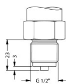
G1/2" EN 837
