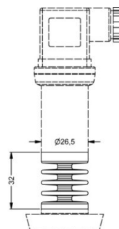
chladič 300 °C
