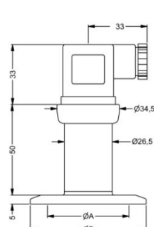
Clamp (DIN 32676) s konektorem ISO 4400
