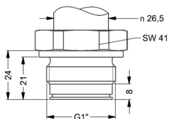
G1" čelní se 2 radiálními o-kroužky ( P_N > 0,25 bar)
