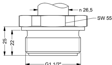
G1 1/2" čelní DIN 3852 10
