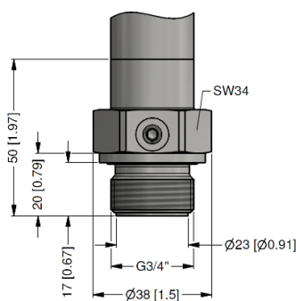
3/4" čelní DIN 3852 s konektorem ISO 4400
