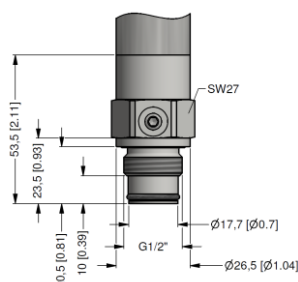
G1/2" čelní s radiálním o-kroužkem 10
