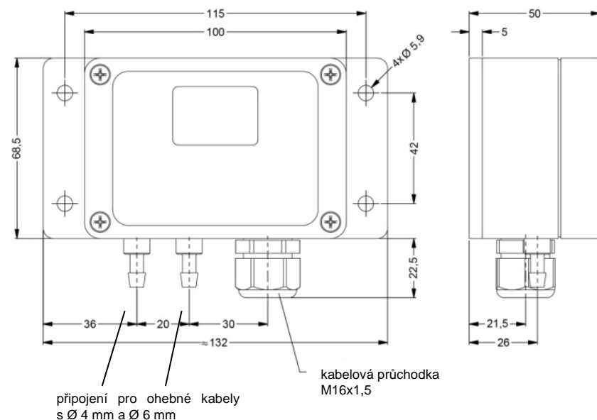
Obr. 3: Rozměry DPS 300 s displejem
