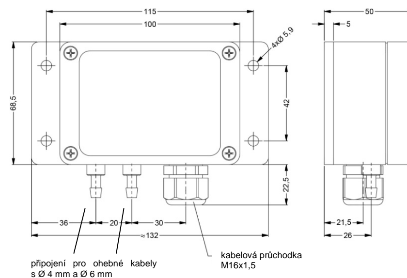
Obr. 4: Rozměry DPS 300 bez displeje
